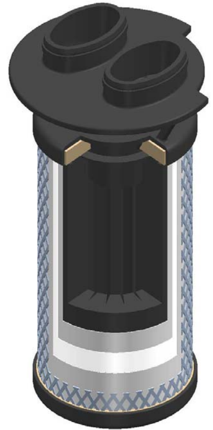
Querschnitt durch den Adsorptionsfilter
