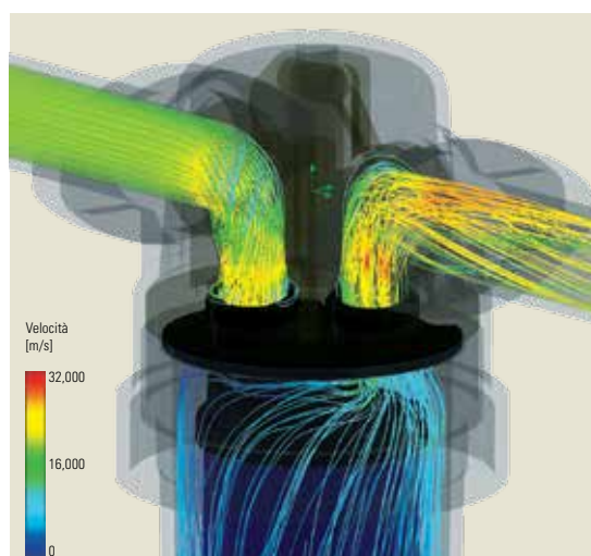
Flusso ottimizzato dell'aria attraverso l'housing
