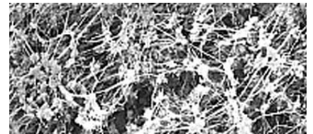
SEM of the Ultrateflomem membrane
